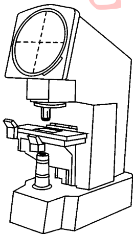
图 1 立式投影仪
